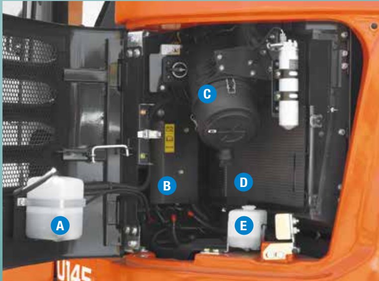
A. Kühlmittelausgleichsbehälter D. Klimaanlage B. Relaiskasten E. Scheibenwaschbehälter C. Luftfilter
